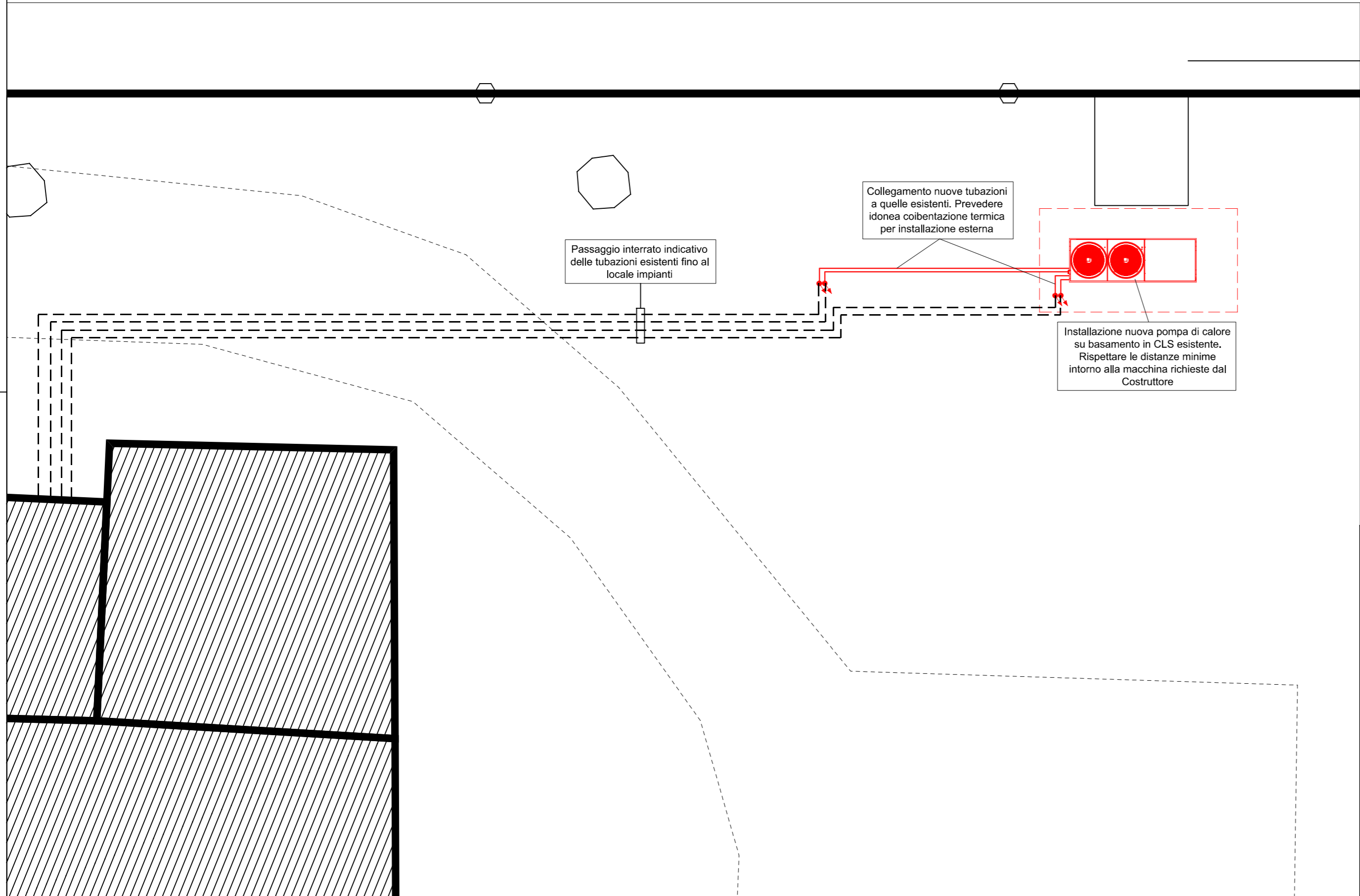
DETTAGLIO PIANTA PORZIONE ESTERNA POSIZIONAMENTO UNITA' POLIVALENTE
