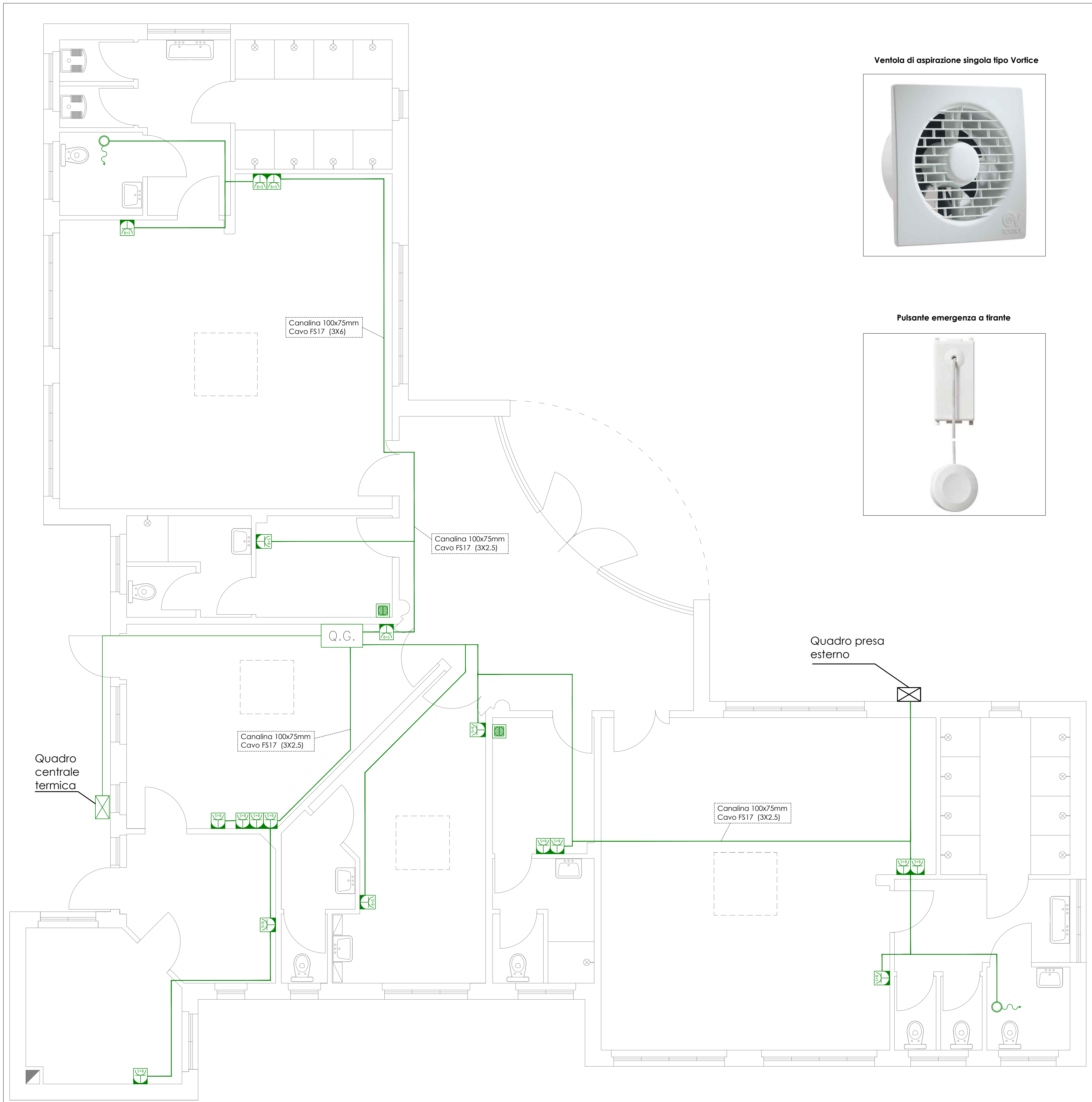
PIANTA IMPIANTO ELETTRICO FORZA PIANO TERRA scala 1:50
