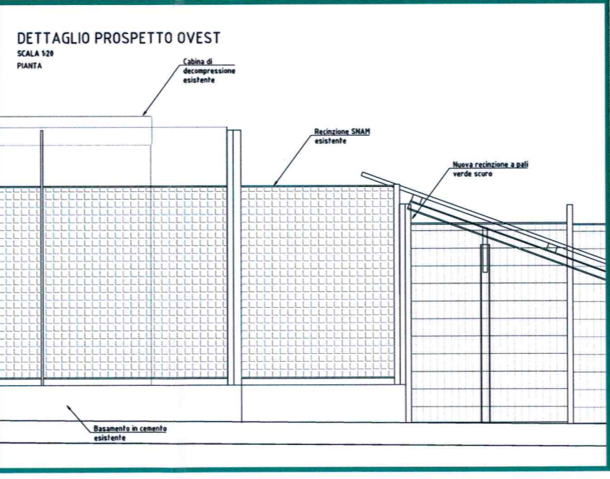
DETTAGLIO 2 RACCORDO TRA RECINZIONE ESISTENTE E NUOVA RECINZIONE CON PALI VERDE SCURO
