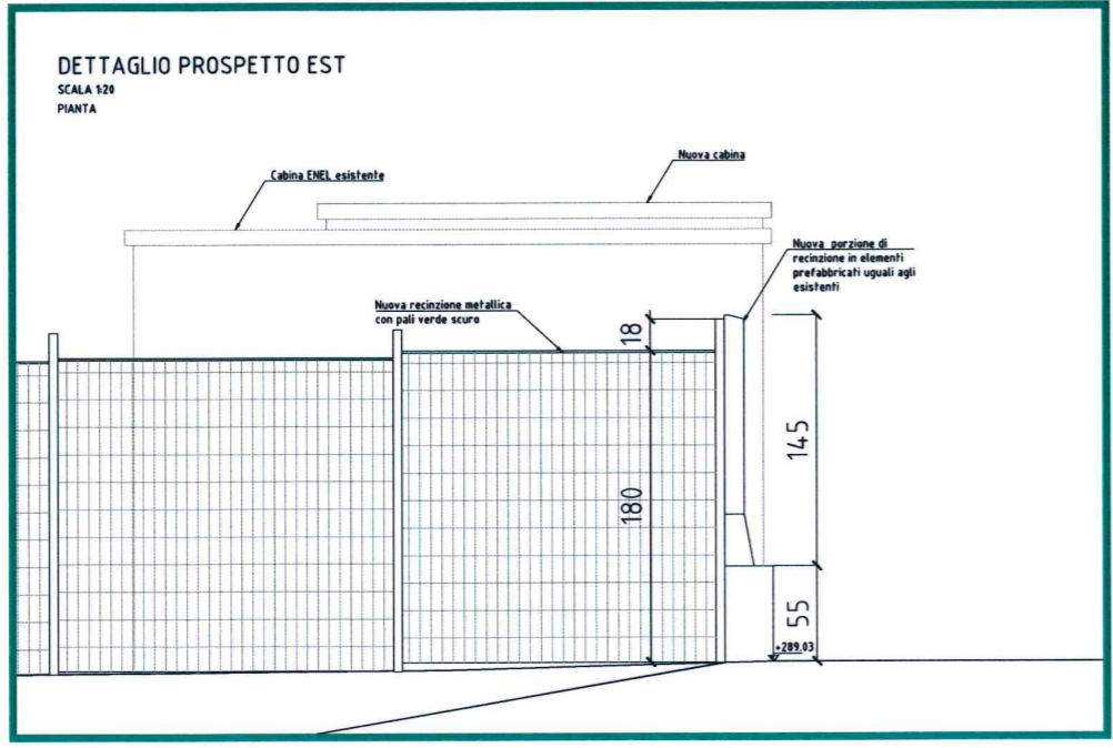
DETTAGLIO 1 RACCORDO TRA RECINZIONE PREFABBRICATA ESISTENTE E NUOVA RECINZIONE CON PALI VERDE SCURO
