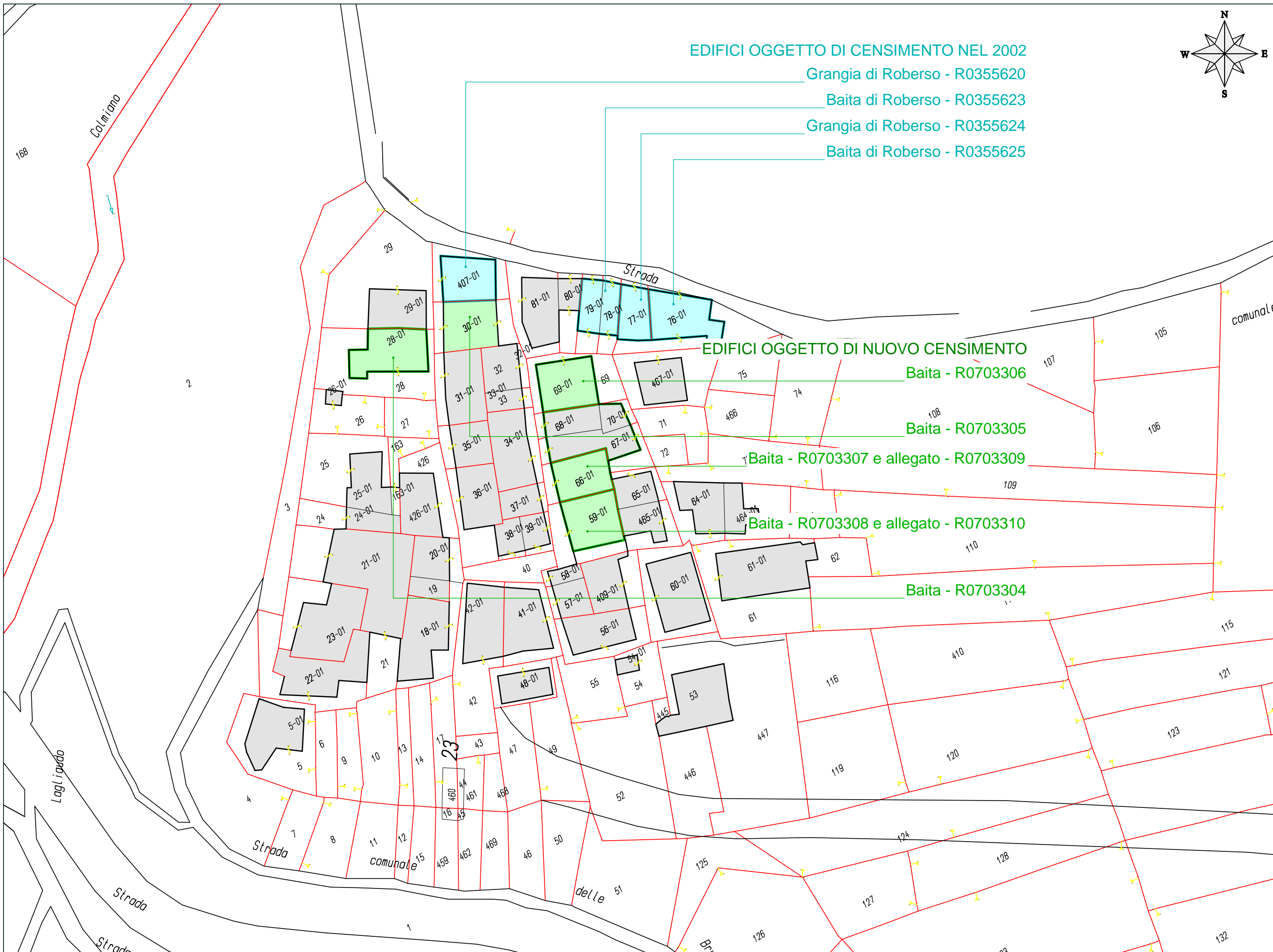
ESTRATTO CATASTALE DI MASSELLO - F. 23 - scala 1:500
